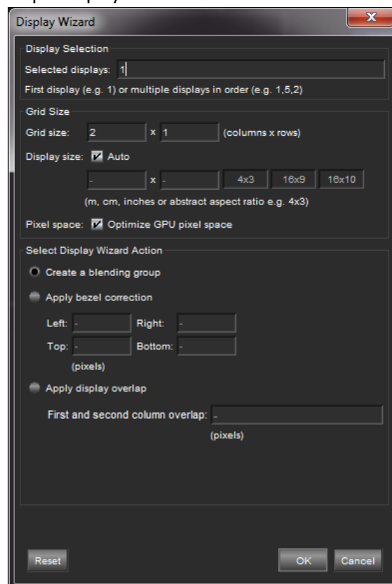
Fig. 63 - Display wizard
