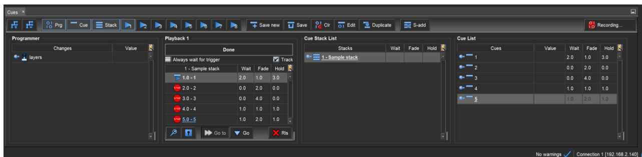
Fig. 92 - Cues panel
